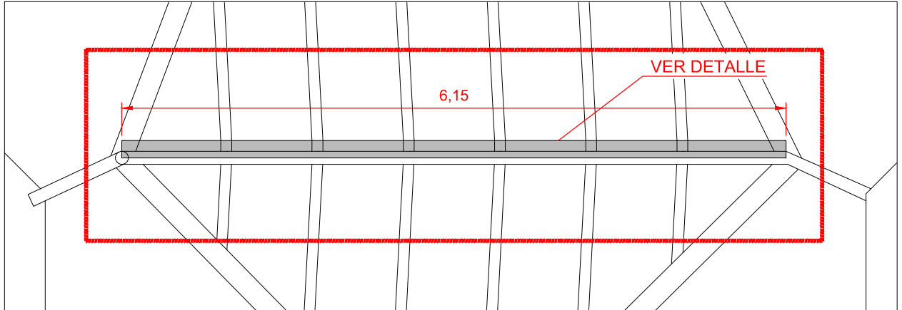
DETALLE DE ZINGUERIA - ESC1:50
