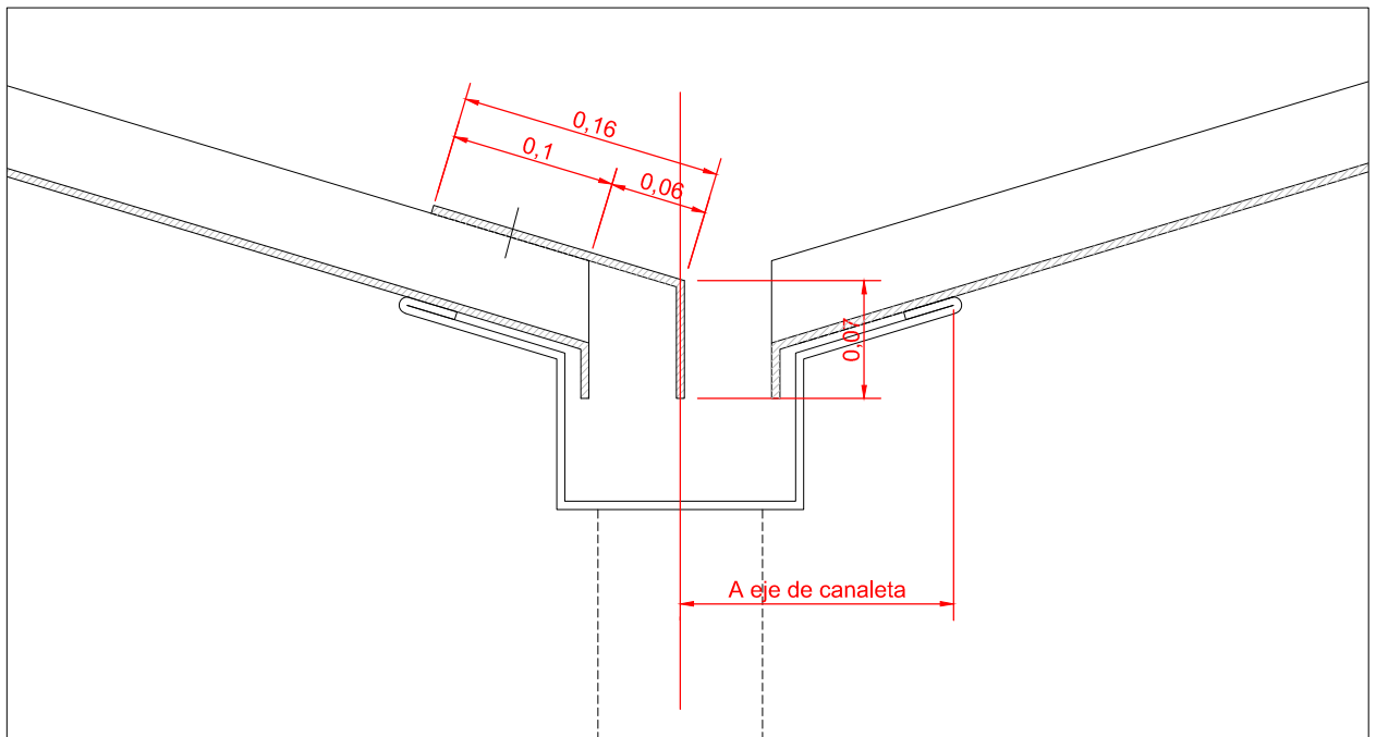
DETALLE DE ZINGUERIA - ESC1:5
